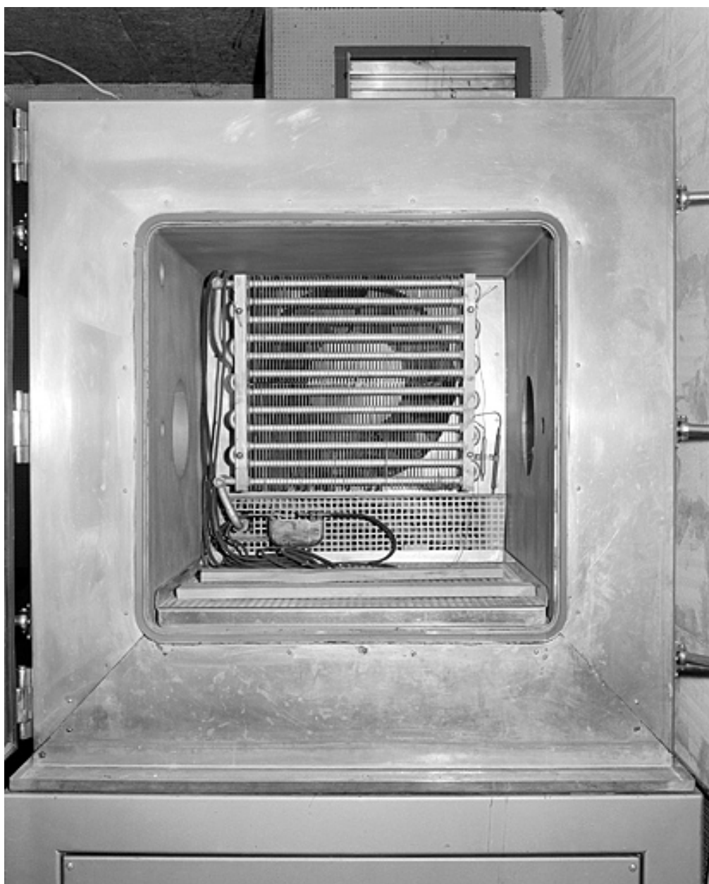
Enceinte d'essais : intérieur.
