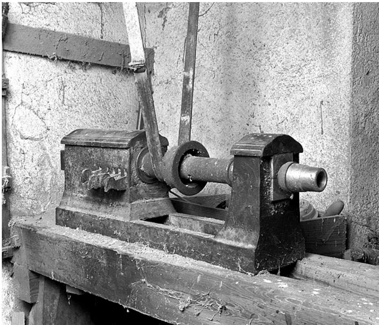
Usine de tableterie (tournerie) Vuillermoz, Vulvoz (au Moulin) : tour à bois Lartaux (Saint-Claude).
