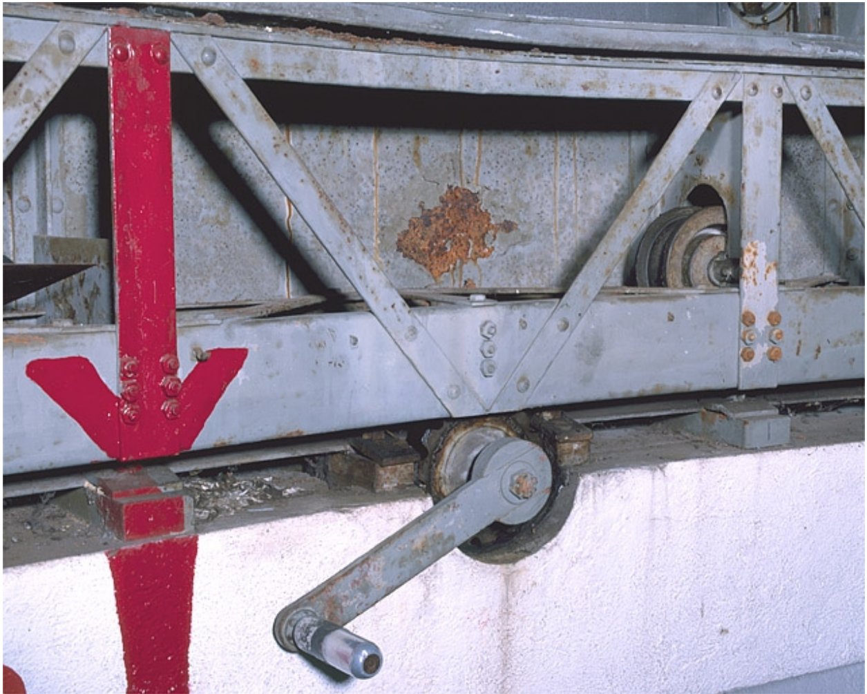
Système de rotation de la coupole : manivelle.
