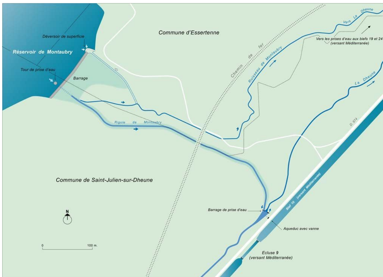
Carte schématique du barrage et de la rigole de Montaubry.
