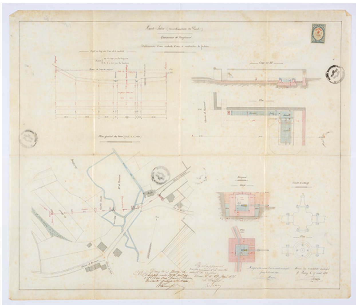
Etablissement d'une conduite d'eau et construction de fontaines, plan général des lieux. [plan, coupes, élévations] 1878
