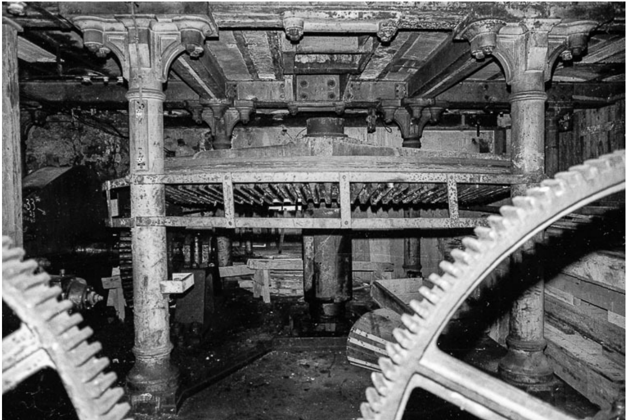
Mécanisme de transmission de la turbine (canal principal) en 1979.
