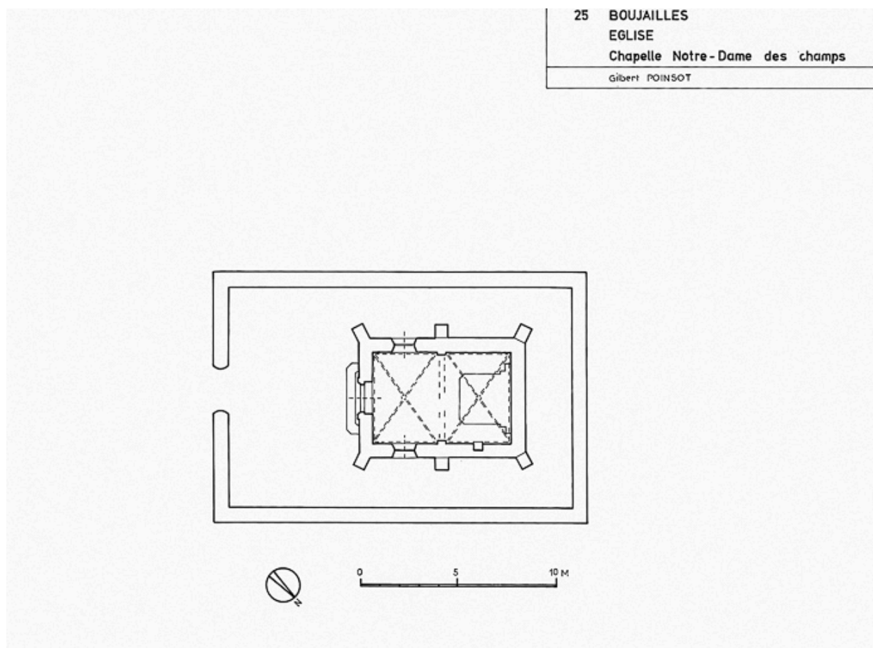
Plan au sol : relevé-croquis G. Poinso, 1975.
