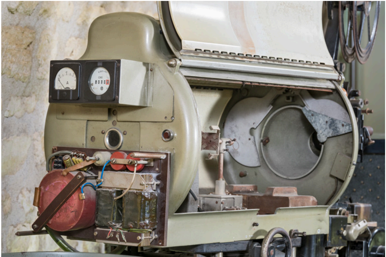
Lanterne Cinemeccanica Zenith VX.
