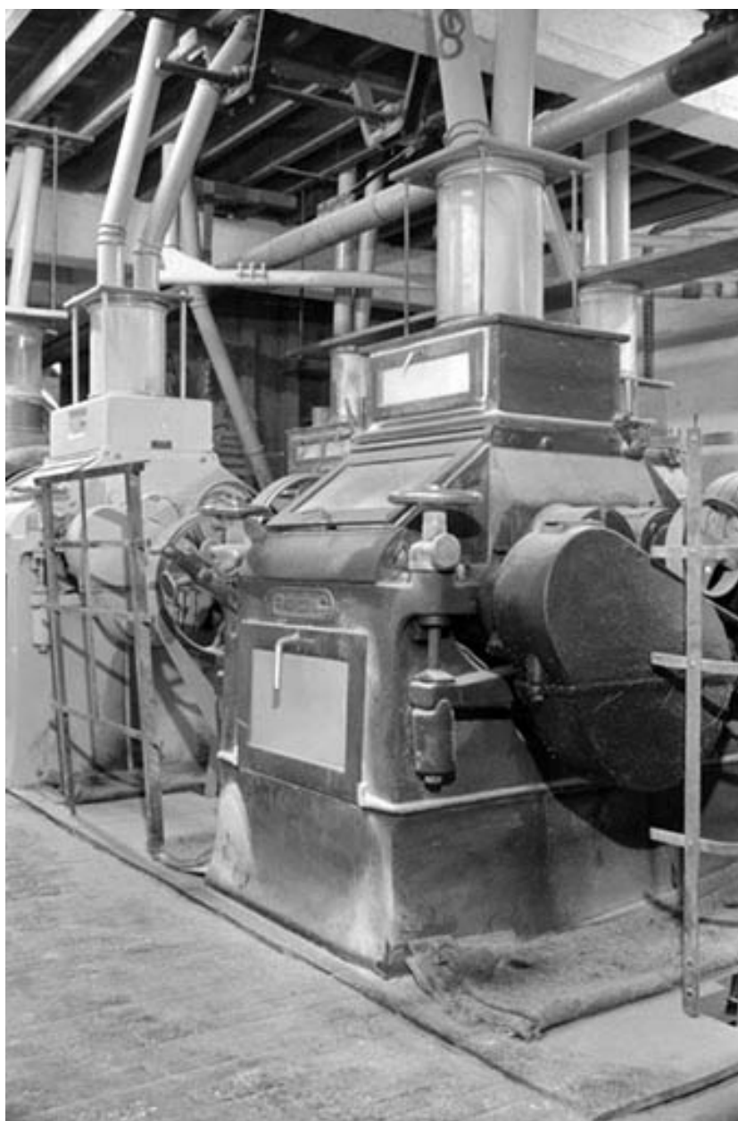
Minoterie, intérieur : appareil à cylindres Buhler.
