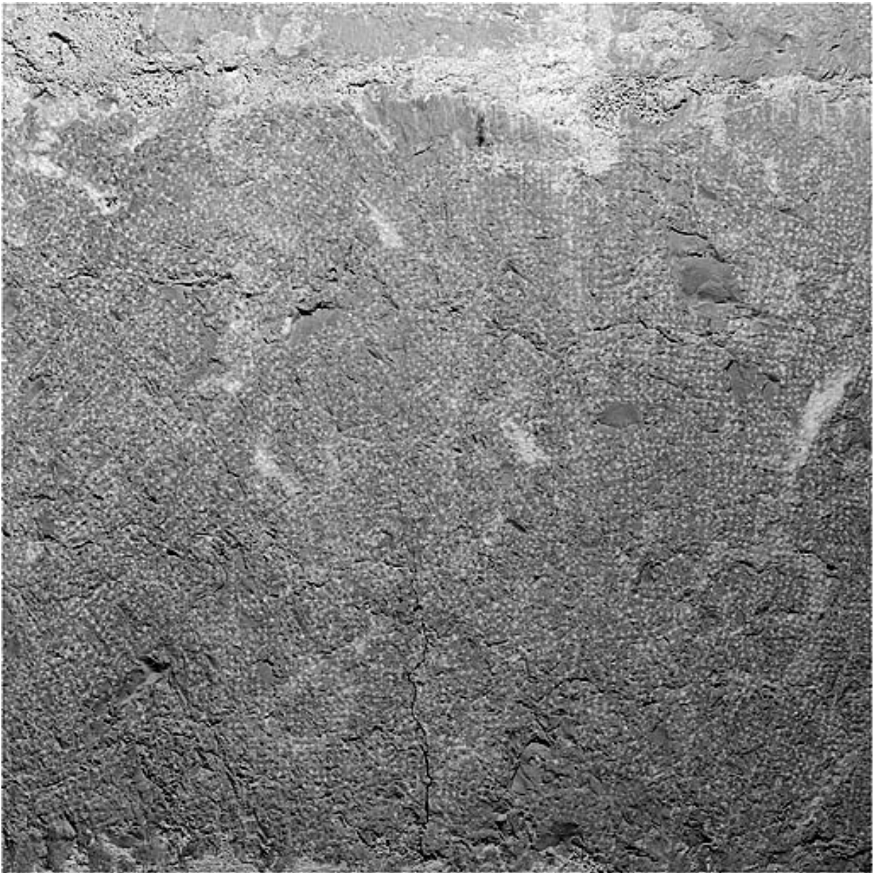
Détail du parement du revers de la façade au nord (traces de boucharde).
