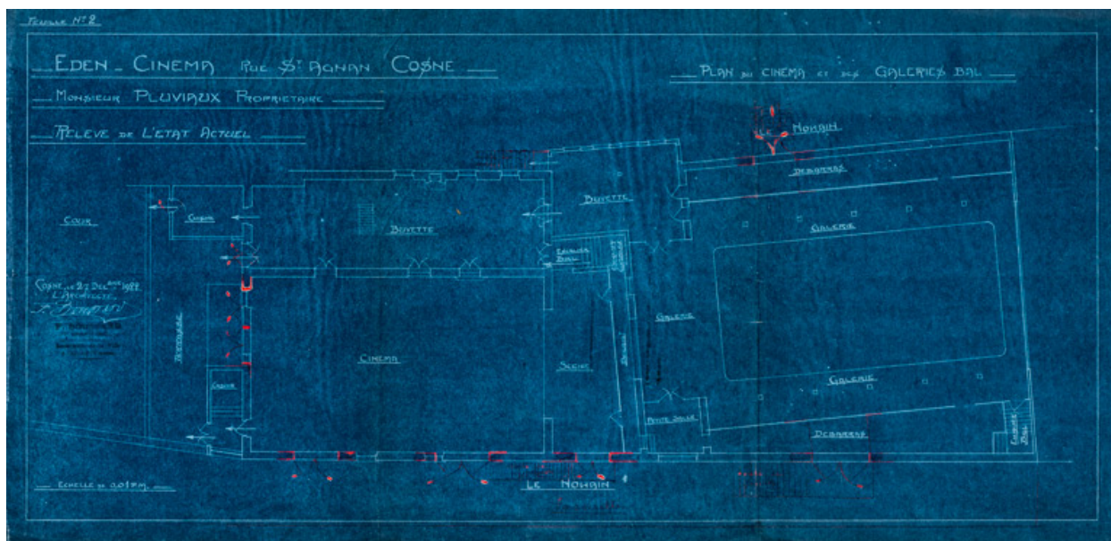
Eden-Cinéma rue St Agnan Cosne. Monsieur Pluviaux propriétaire. Relevé de l'état actuel. Plan du cinéma et des galeries bal. 1922.
