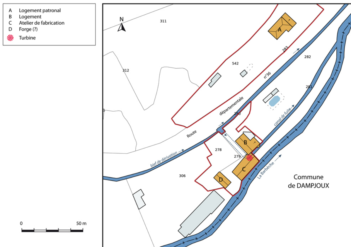
Plan-masse et de situation, section B.
