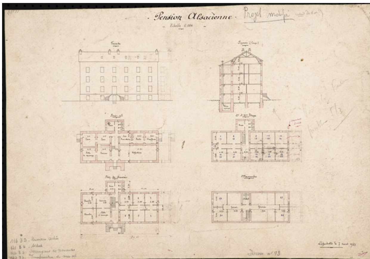
Pension alsacienne. Plans, coupes, élévation, échelle 1/250, Lafeschotte, 7 août 1923.
