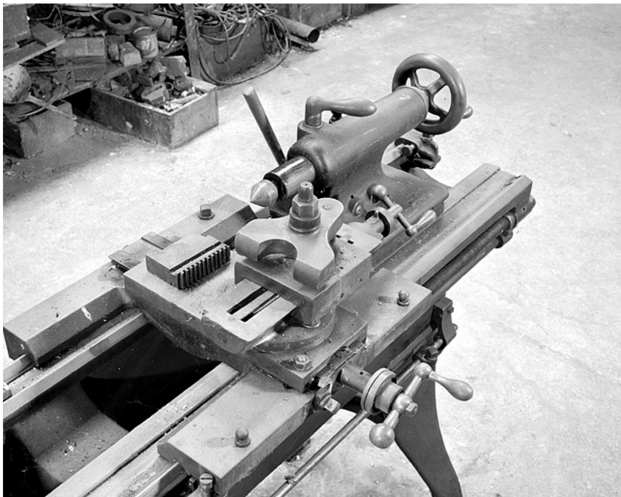
Détail du traînard et de la poupée mobile.
