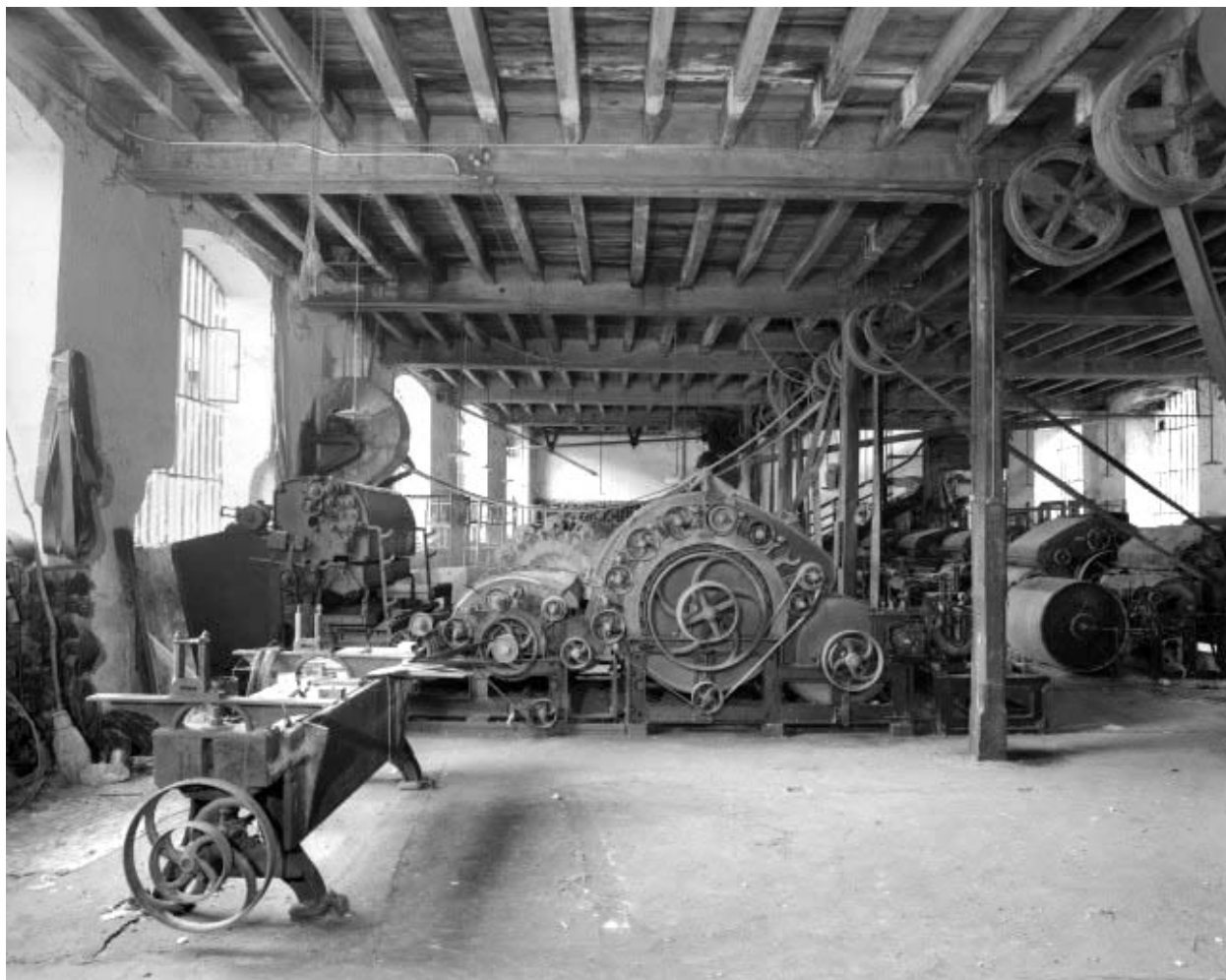
Vue d'ensemble : face latérale droite.
