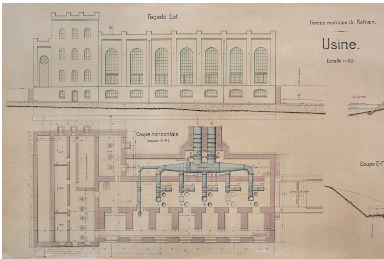
Forces motrices du Refrain. Usine [détail : plan du soubassement et élévation orientale], 1908.
