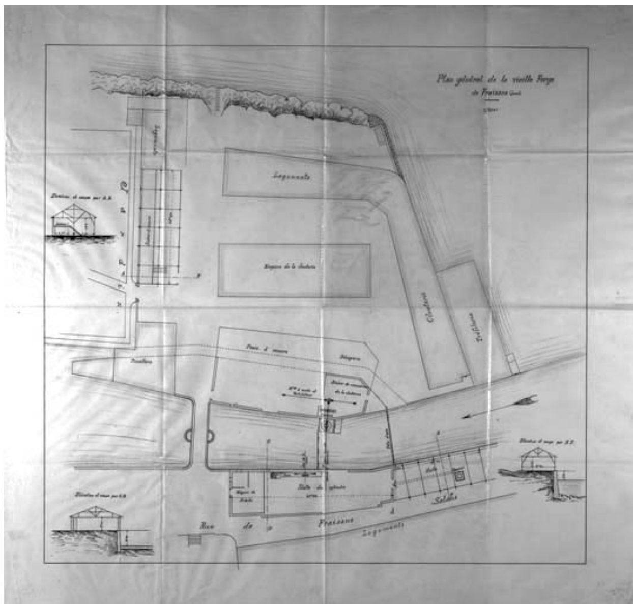
Plan général de la Vieille Forge de Fraisans (Jura).
