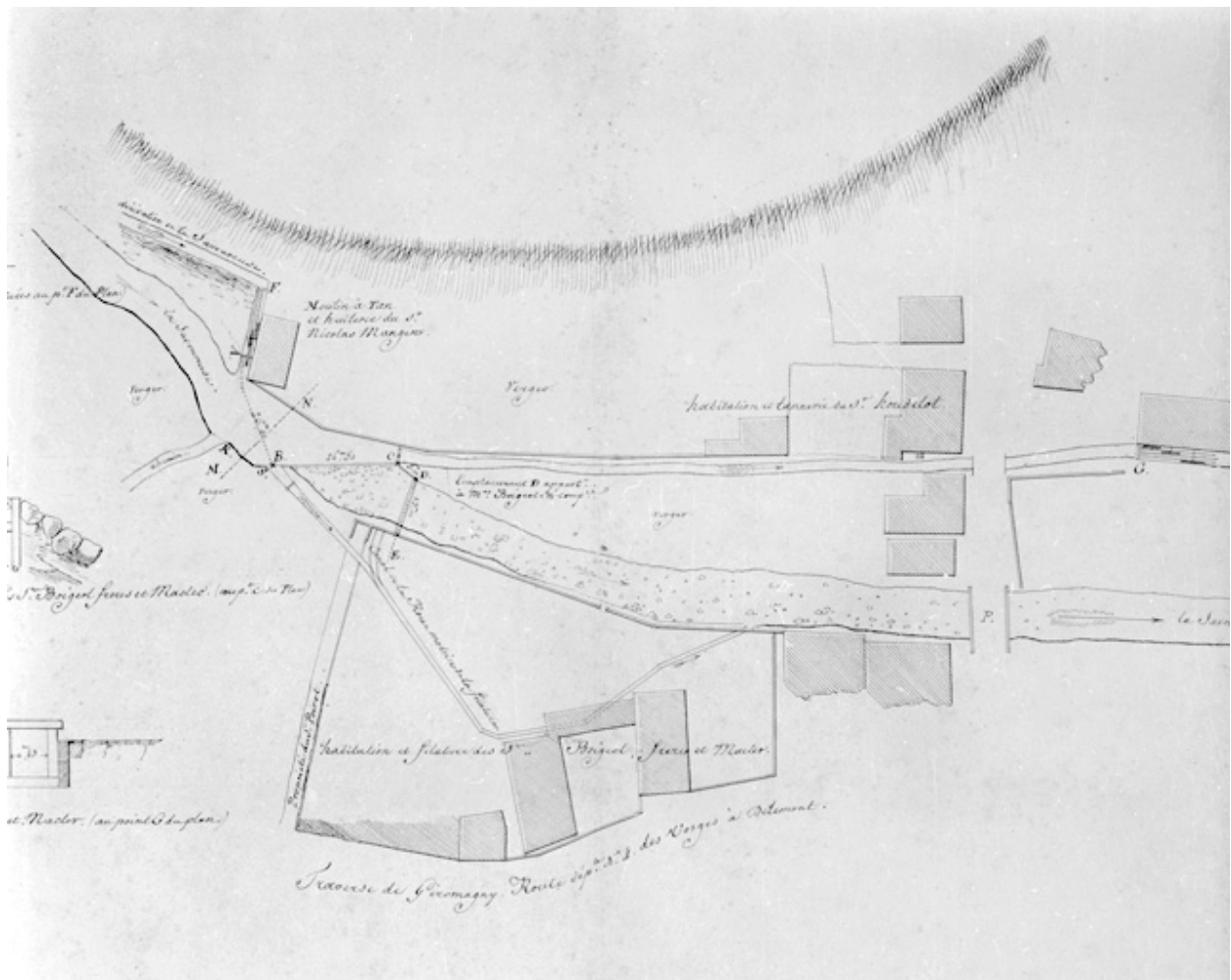
Plan-masse et de situation de la filature Boigeol frères et Macler.
