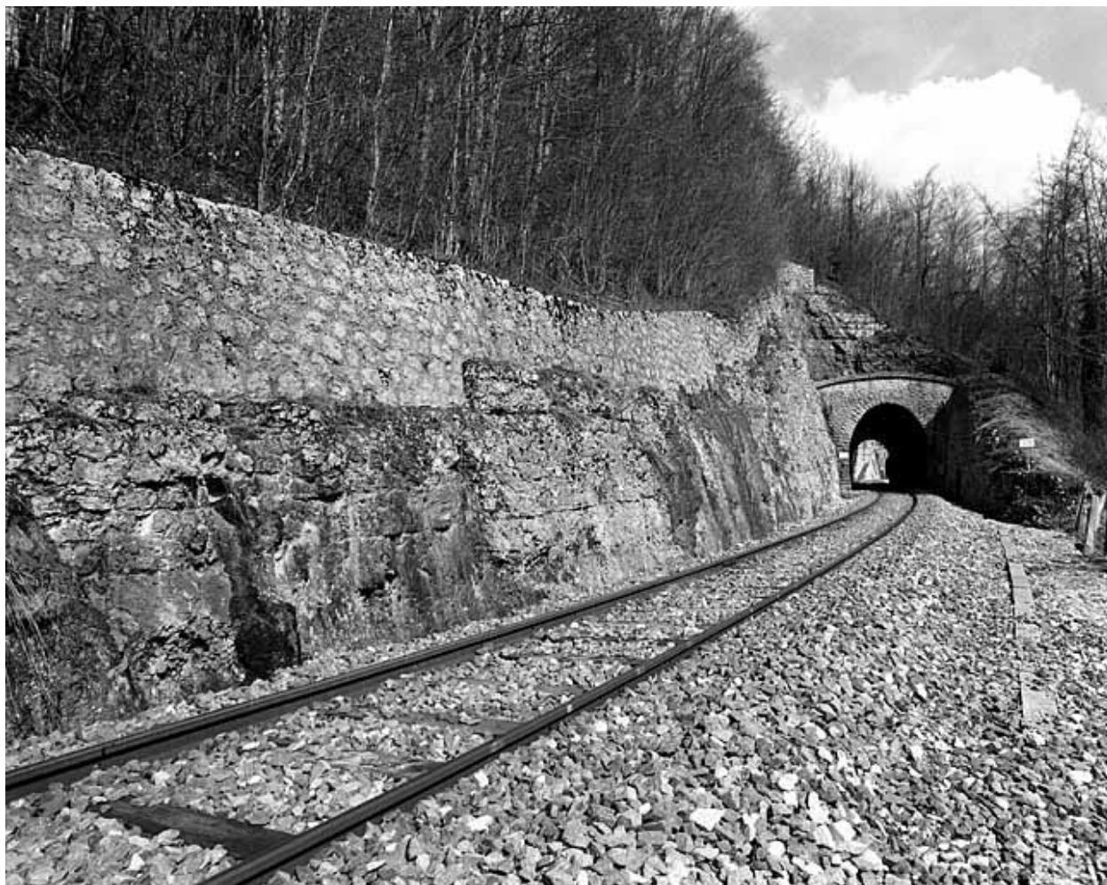
Tunnel de Tancua : vue d'ensemble, côté La Cluse (sud).
