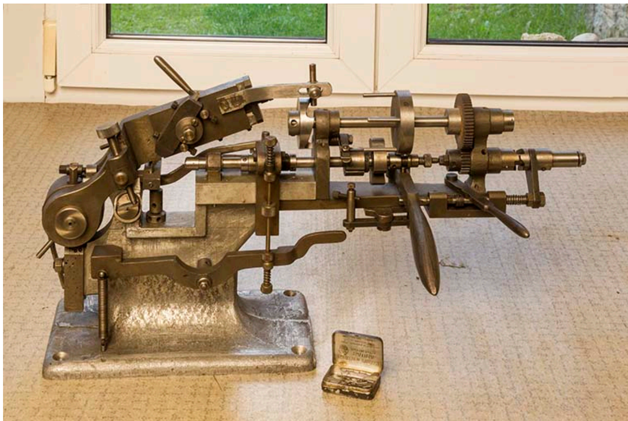
Machine à fabriquer les tire-nerfs pour dentiste (atelier de construction mécanique Berçot puis Roch, Maïche).
