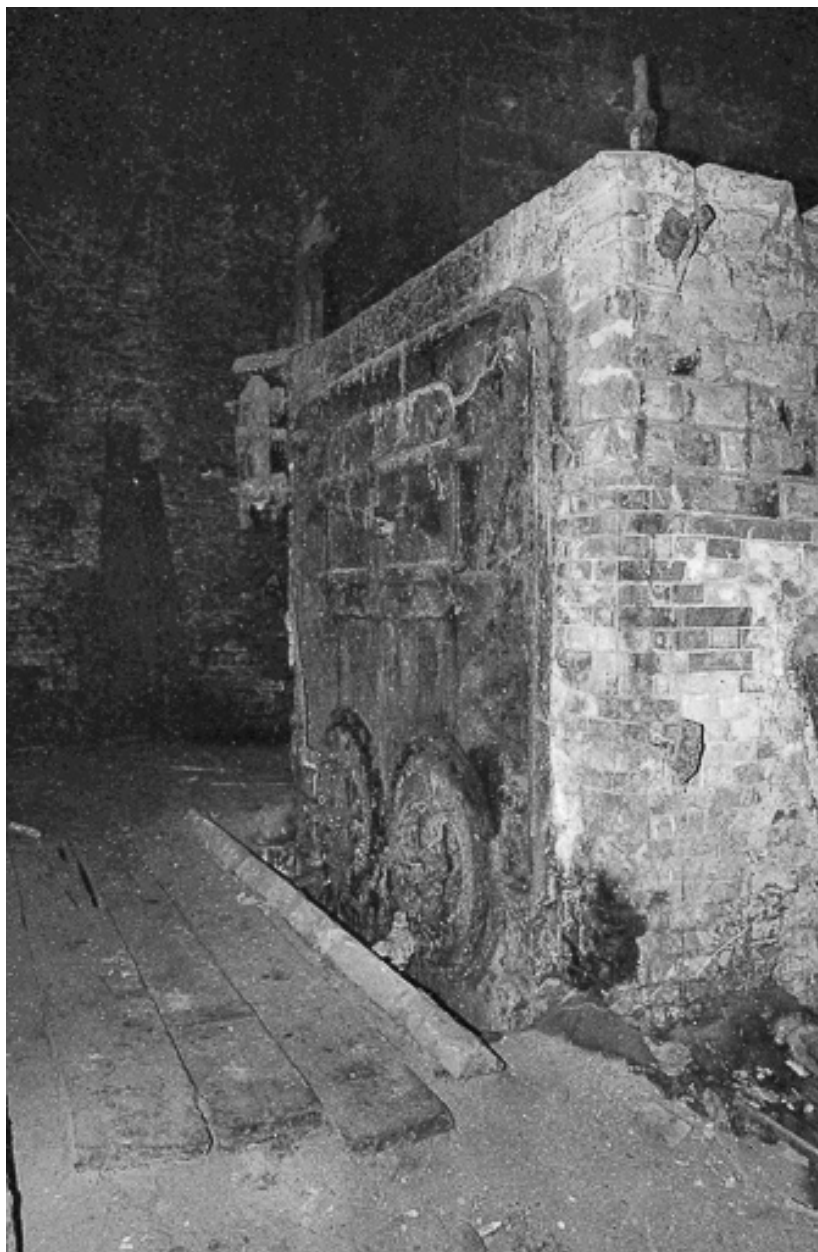
Chaudière de machine à vapeur située à la base du haut fourneau en 1979.
