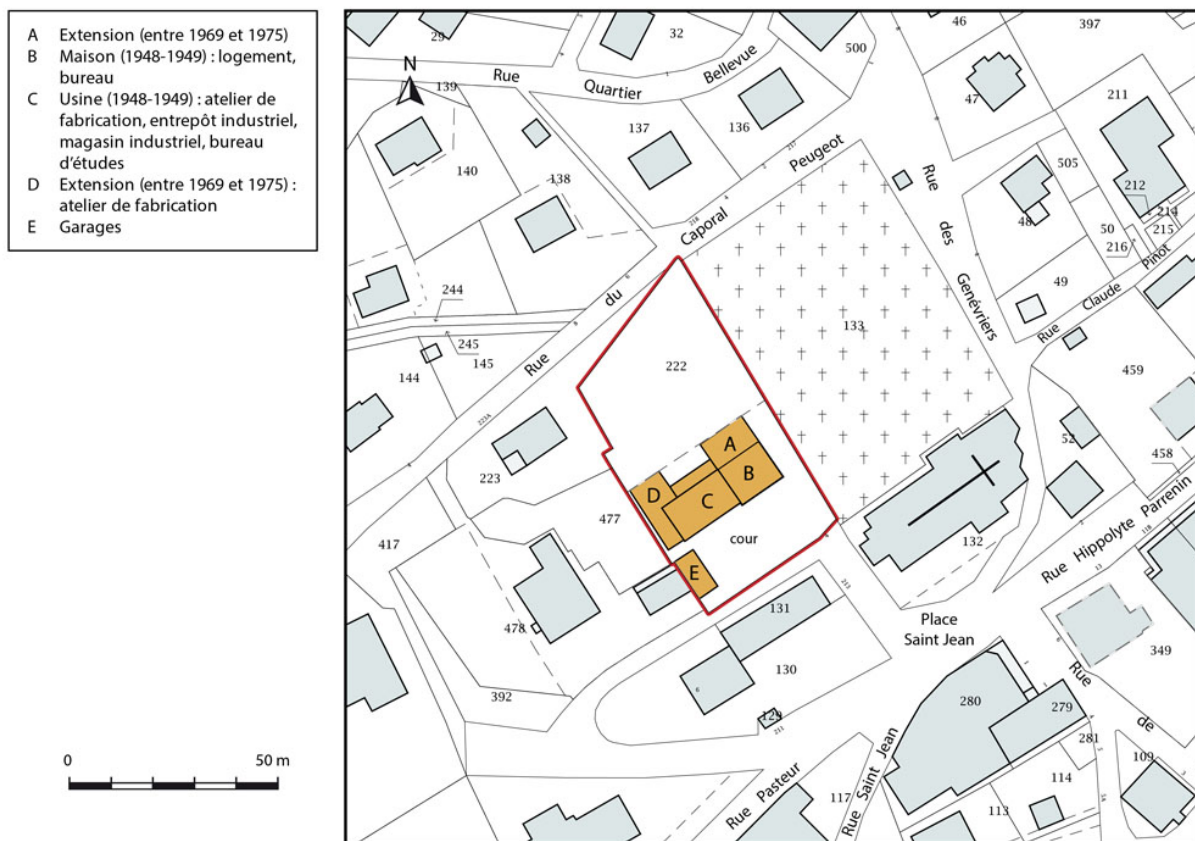
Plan-masse et de situation, avec datation.
