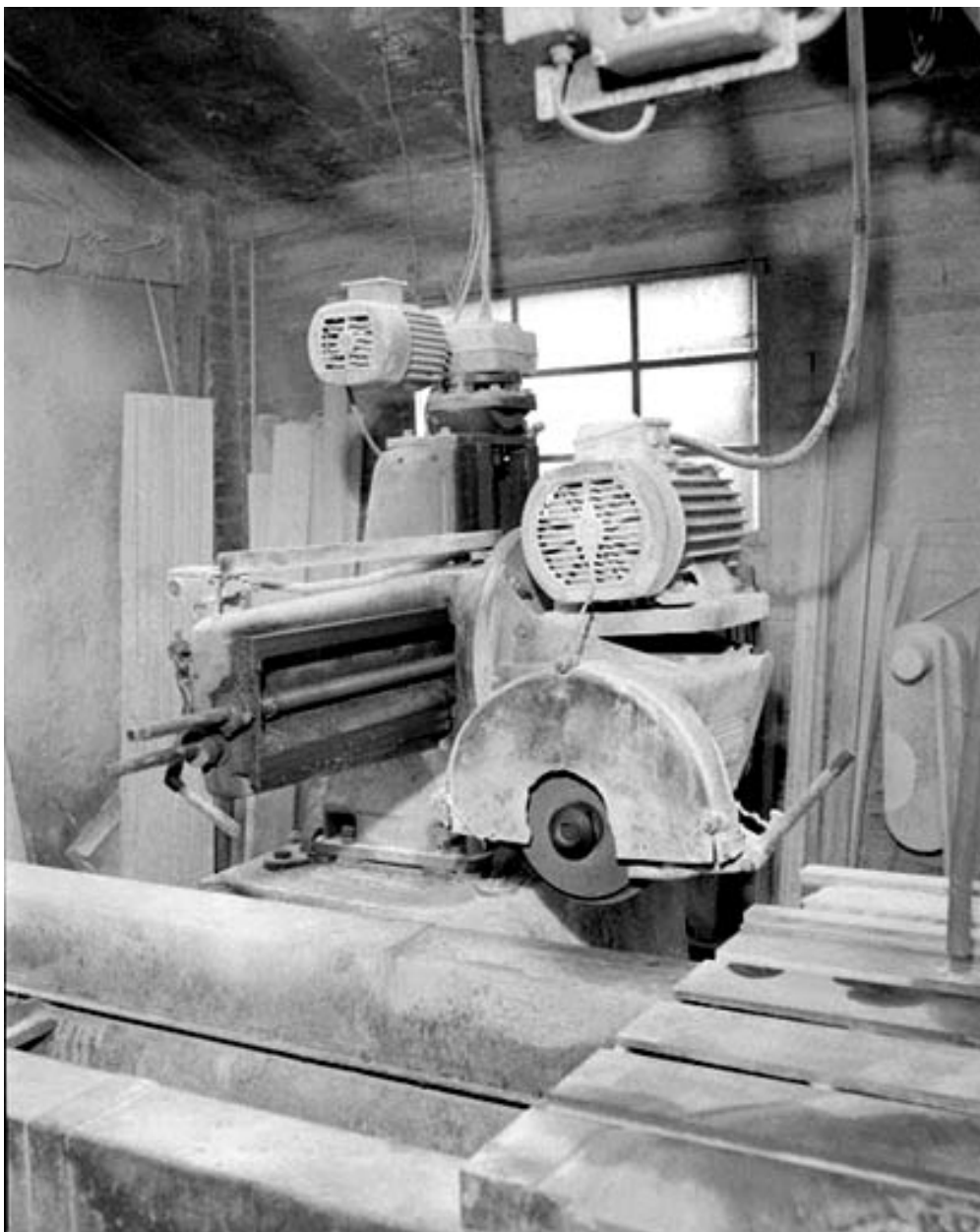
Débiteuse-moulreuseuse sud : bâti vertical, moteur et toupie.
