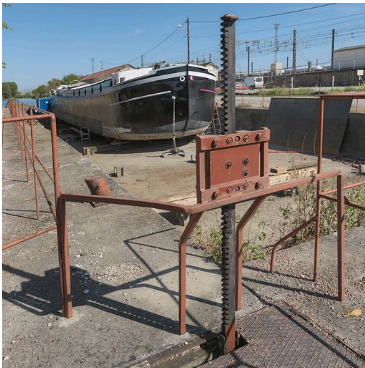
La cale sèche. Détail des vannes.
