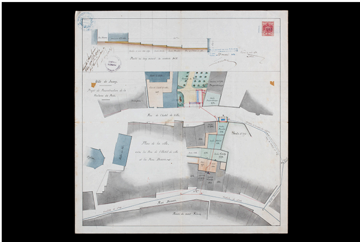
Plan projeté de l'adduction en eau de la fontaine-lavoir des Rois de Jussey, 30 avril 1870.
