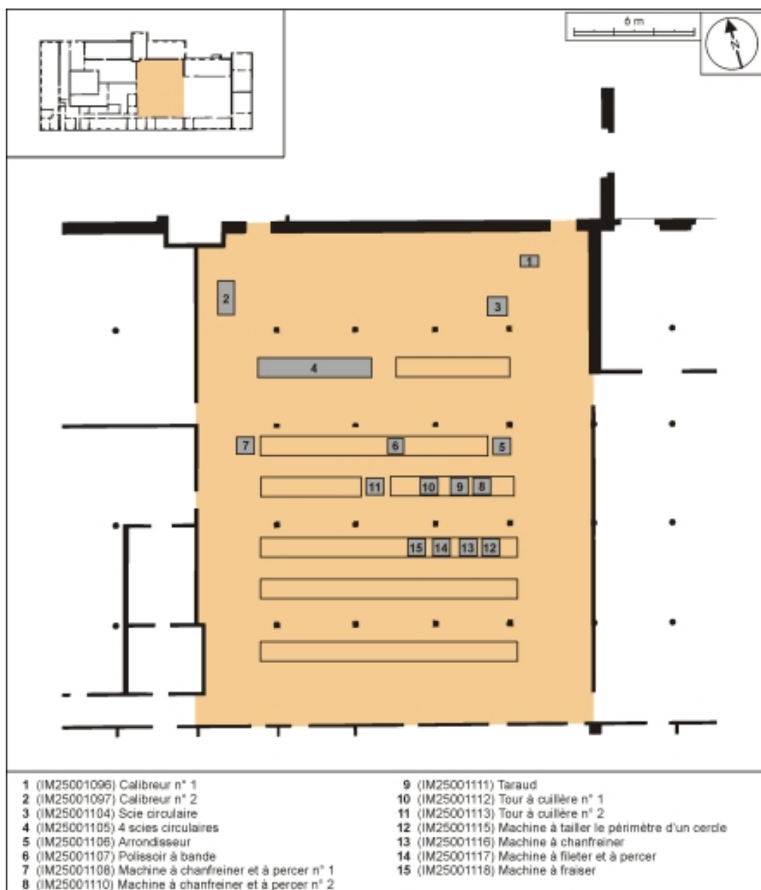
Plan de localisation des machines de la ligne de fabrication des têtes de pipe en merisier.
