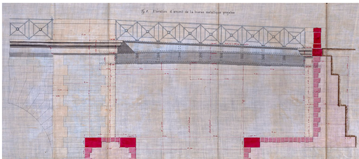
Construction de la partie métallique de la travée marinière du pont de Gray - Plan, élévation, coupes et détails (1882).
