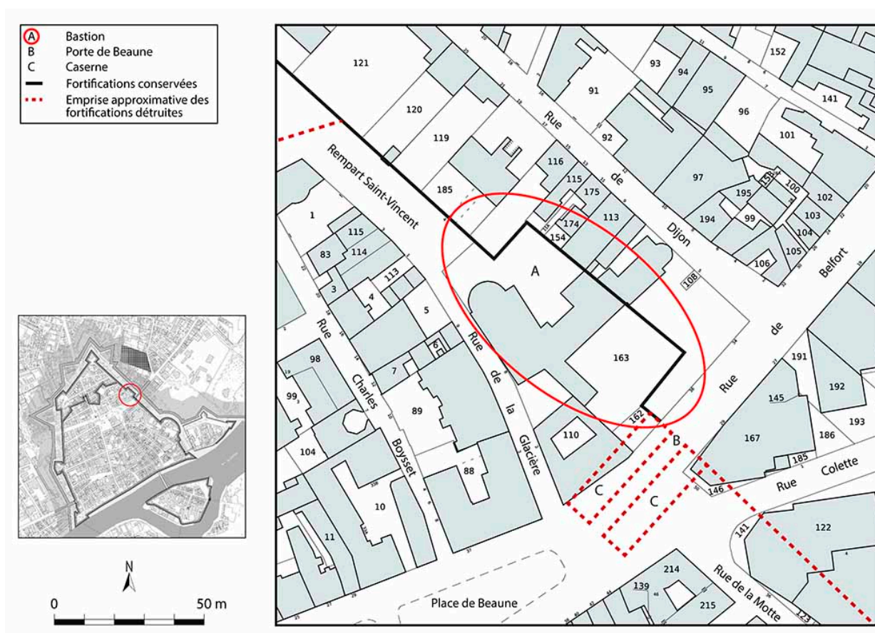
Plan-masse et de situation. Extrait du plan cadastral, 2025, 1/1 000.
