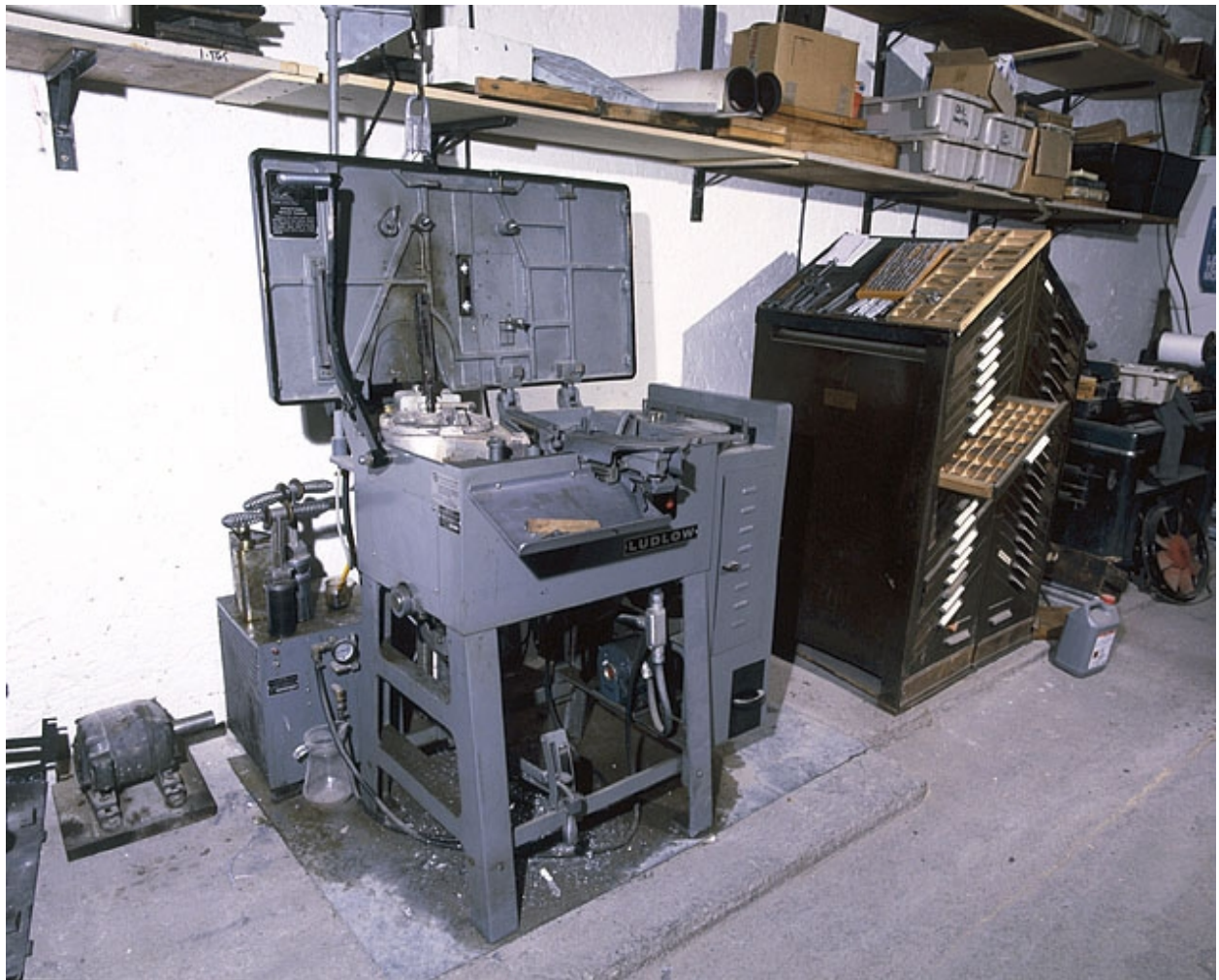
Fondeuse de lignes-blocs et 2 rangs à pupitre.
