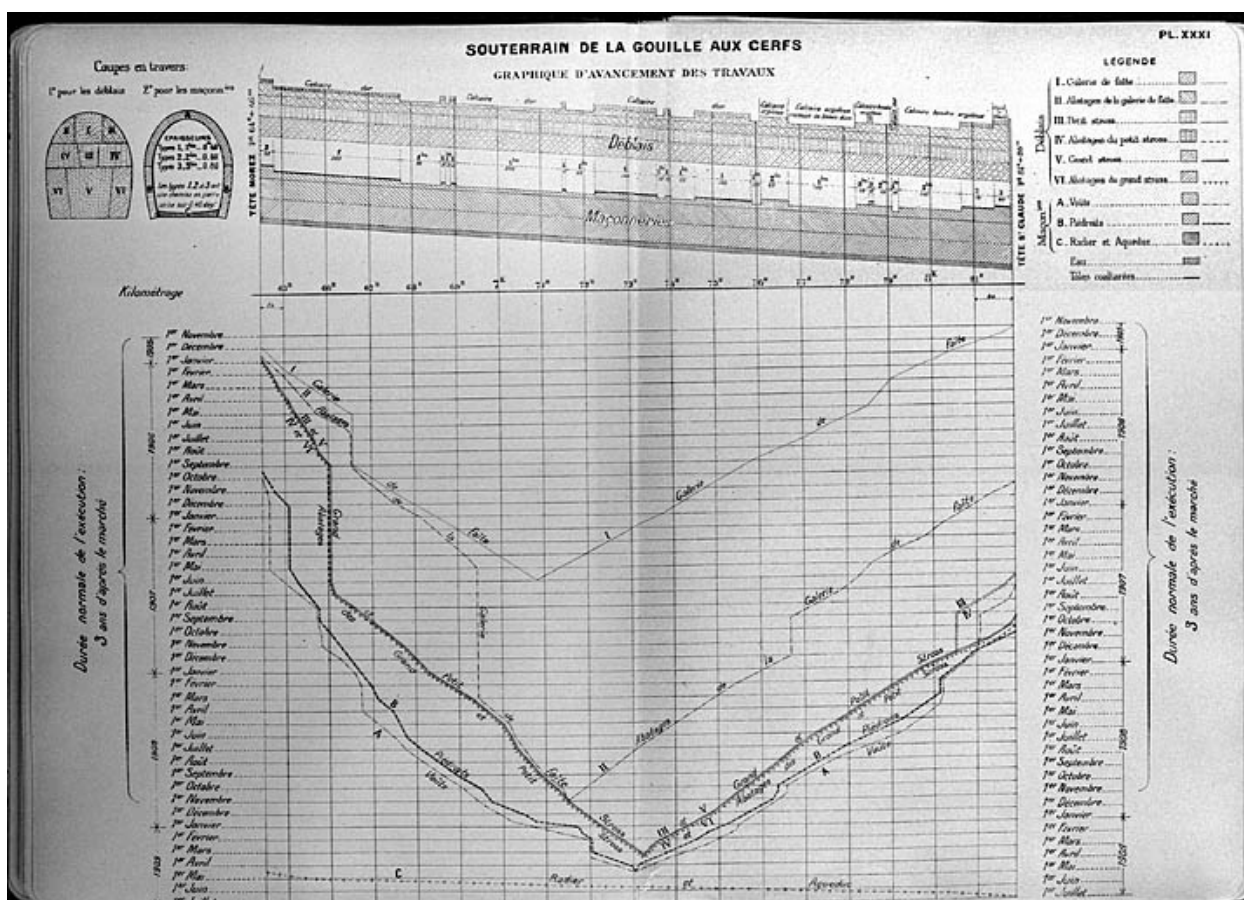
Souterrain de la Gouille aux Cerfs. Graphique d'avancement des travaux, [1919].
