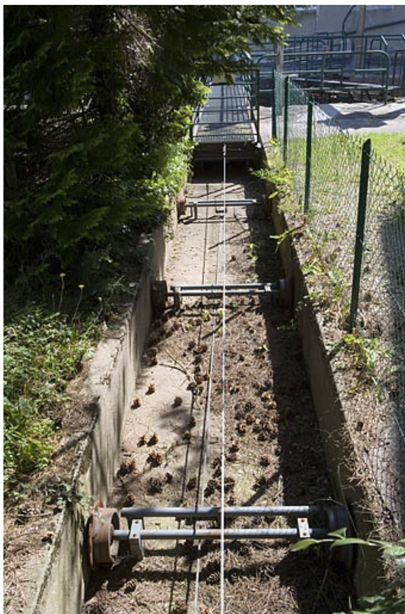
Système d'entraînement de la passerelle.
