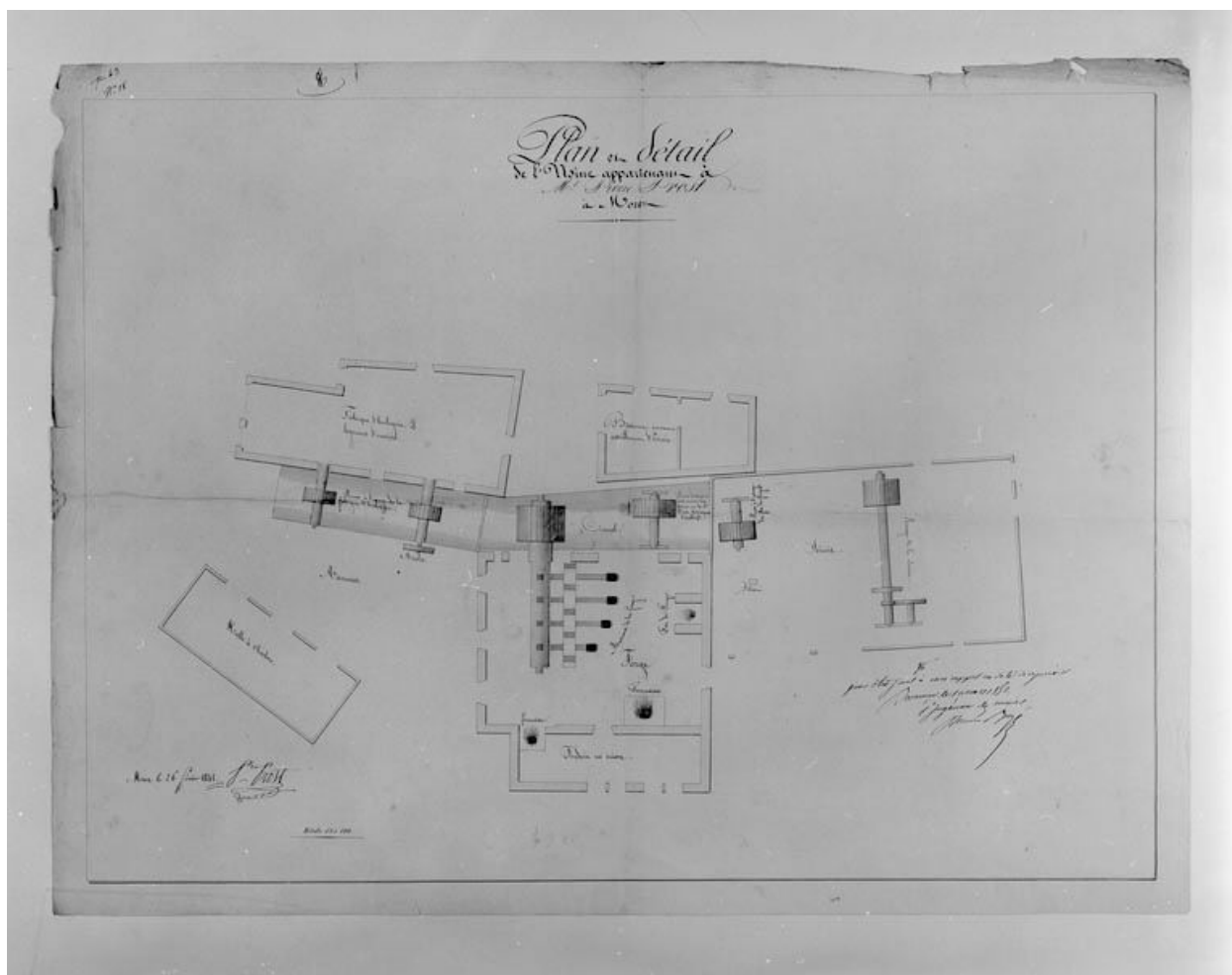
Plan de détail de l'usine appartenant à M. Pierre Prost à Morez. Dessin, 1841. Echelle 1:100.
