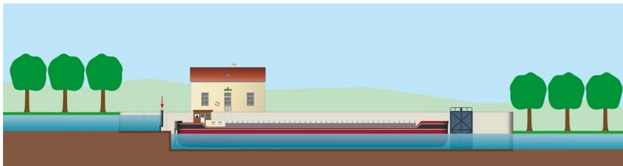
Schéma d'éclusement d'un bateau avalant, étape 8.
