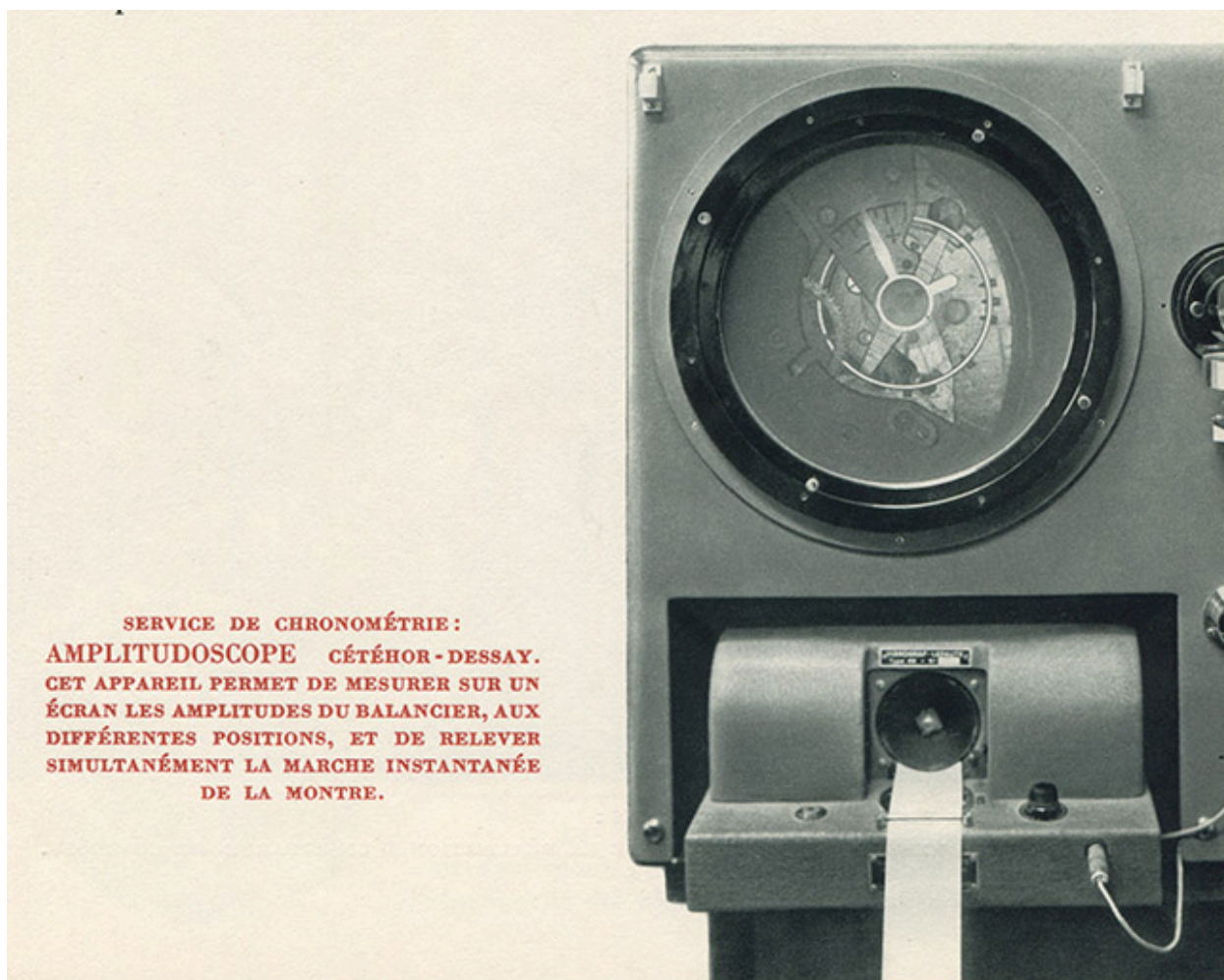
Service de chronométrie. Amplitudoscope, 1955.
