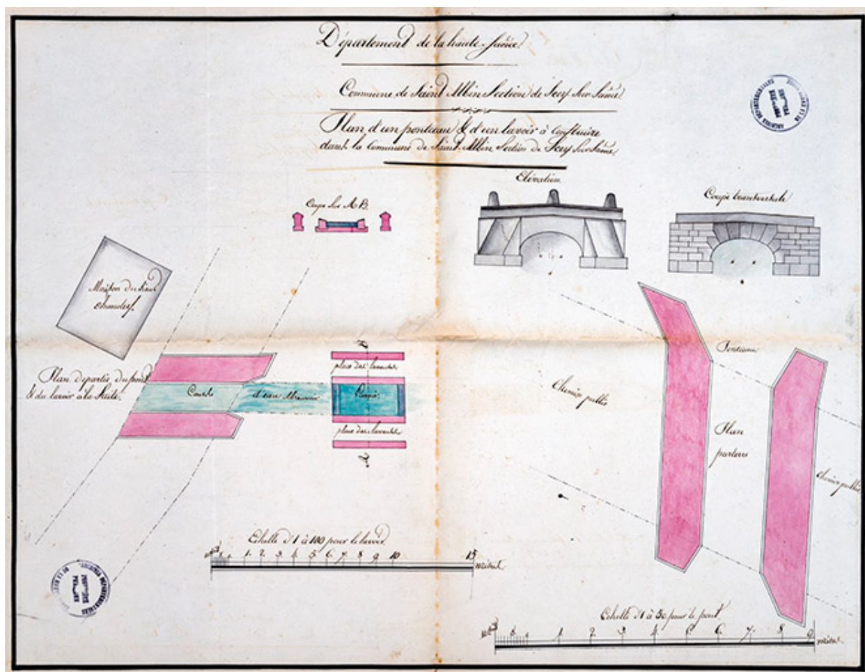
Plan d'un pontceau et d'un abreuvoir à construire dans la commune de Saint-Albin section de Scey-sur-Saône. [1822].
