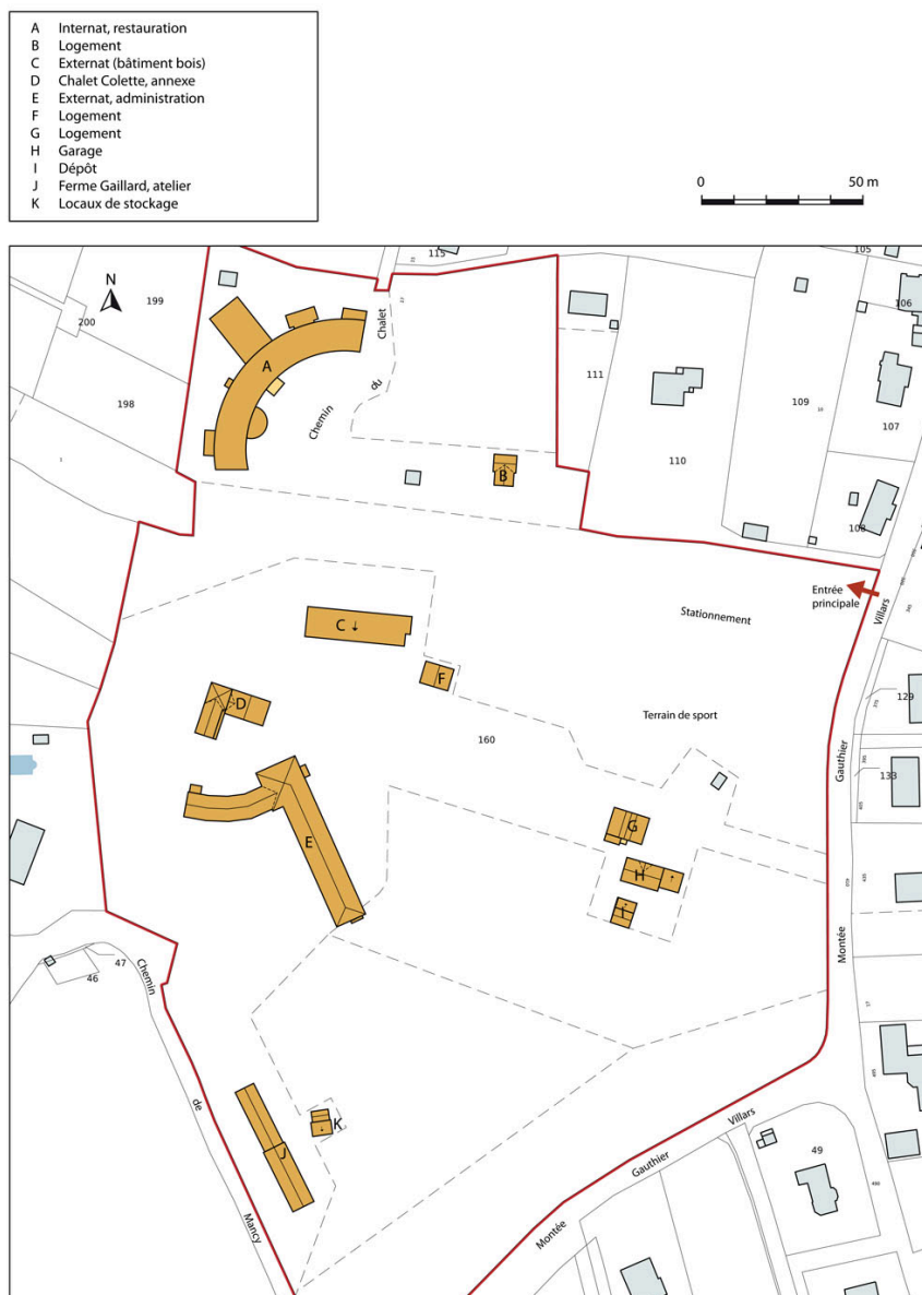
PLan-masse et situation. Extrait du plan cadastral, 2011, section BD, échelle 1/1 500.
