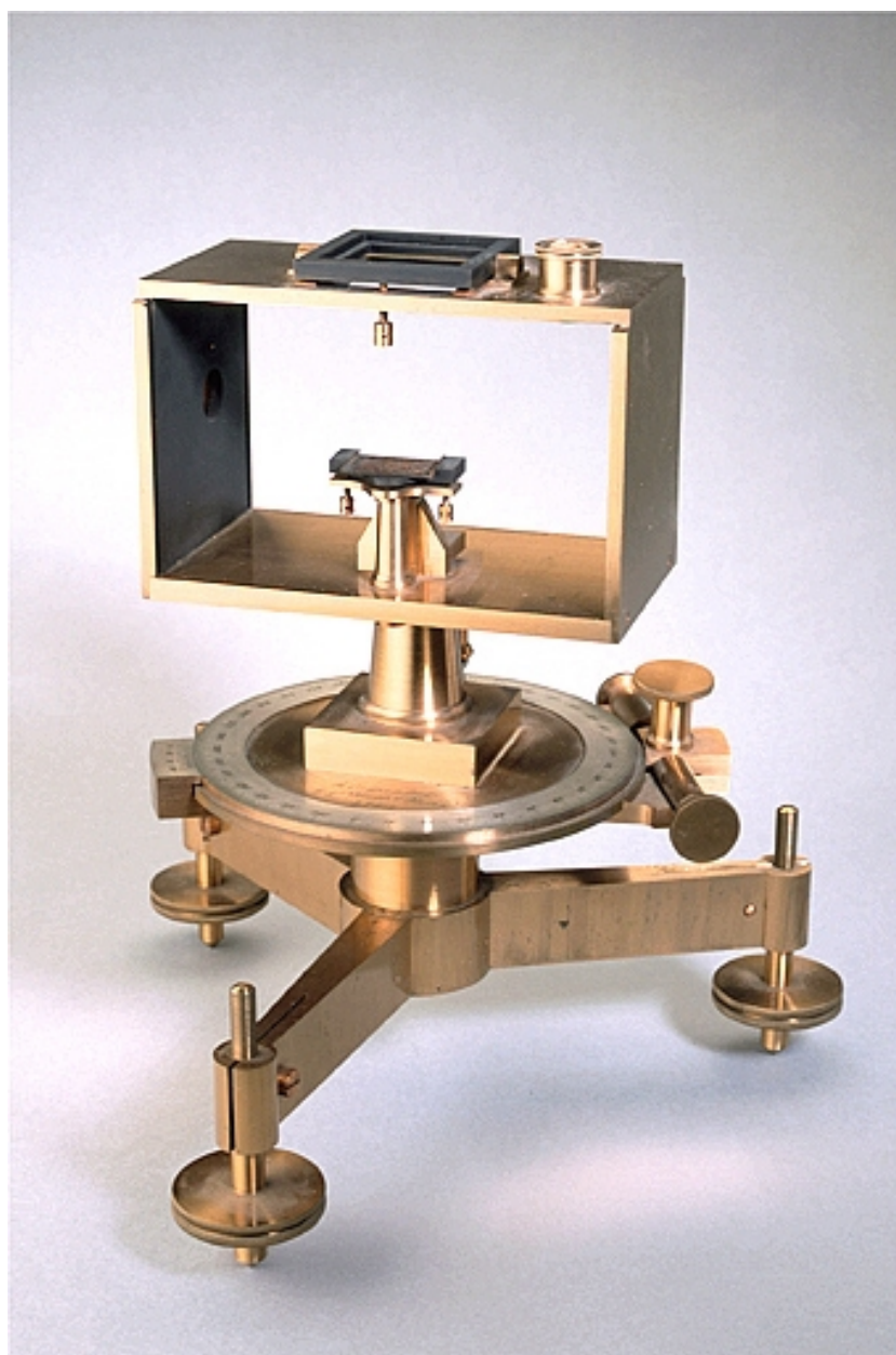
Balance magnétique de Mascart.
