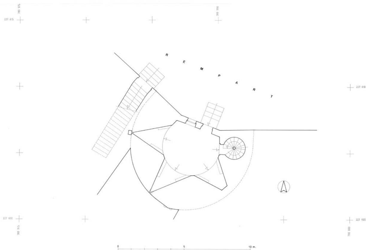
Tour des Cordeliers. Plan du deuxième niveau.
