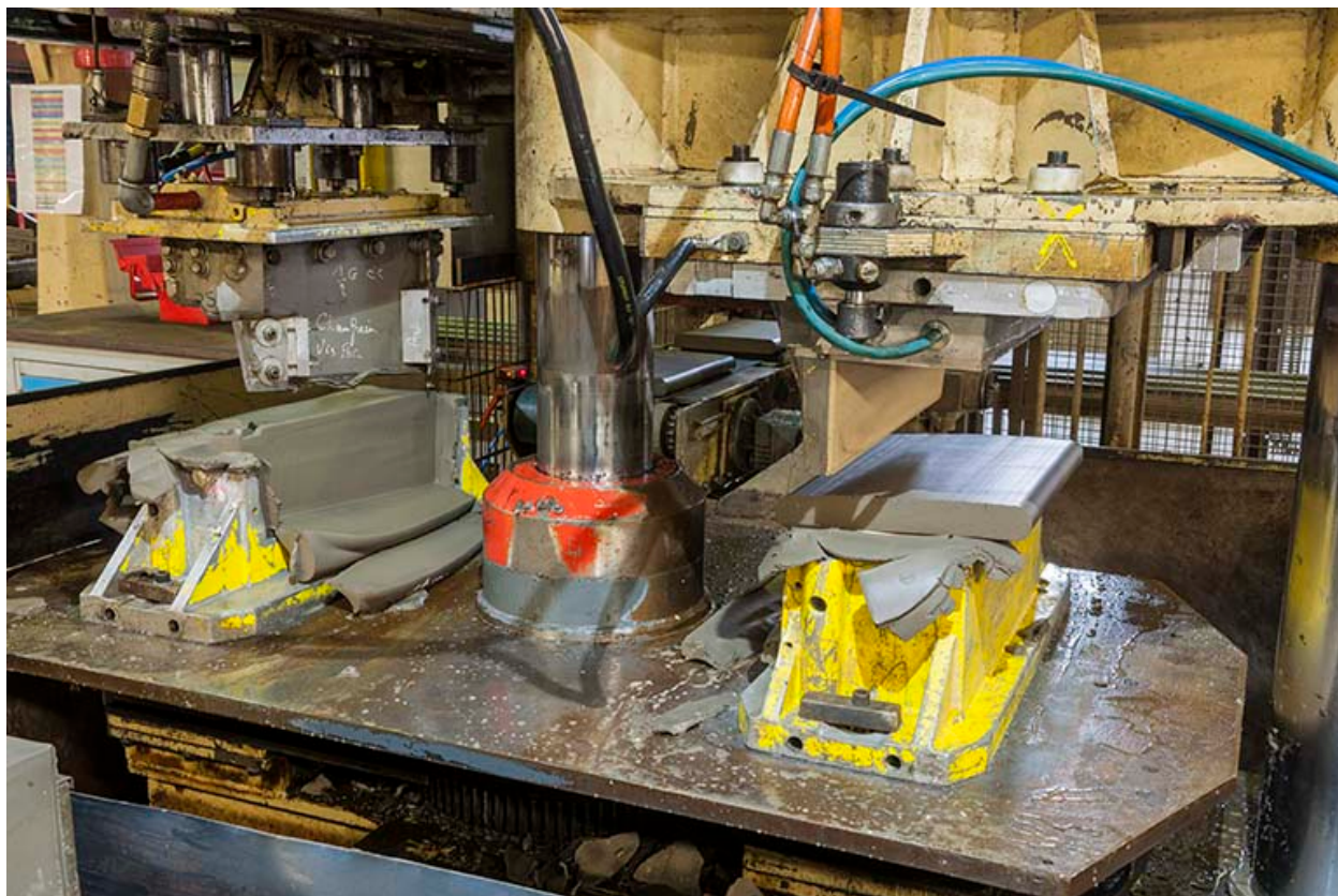
Unité de fabrication dite UL 3. Détail de la machine de pressage (deux têtes).
