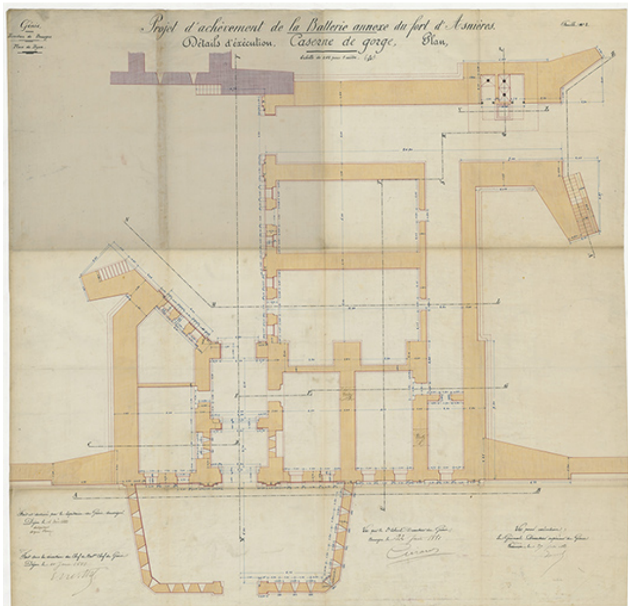
Projets d'achèvement de la batterie annexe du fort d'Asnières. Détails d'exécution, caserne de gorge, plan. 1881.
