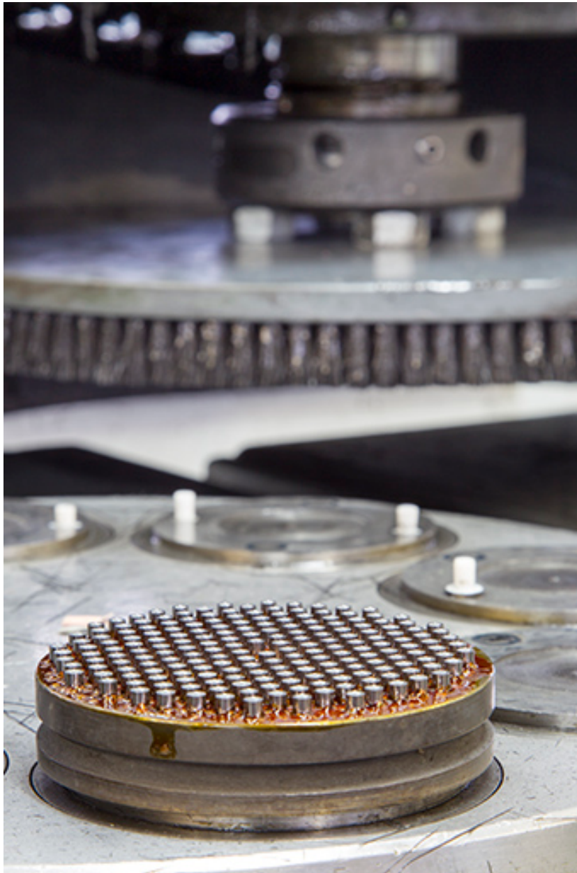
Atelier de polissage : plot monté sur une machine à polir à brosse.
