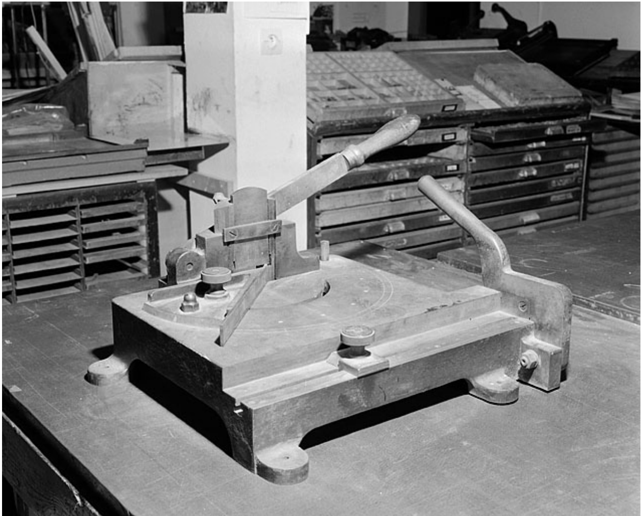
Vue d'ensemble d'un coupleur-biseautier. "Couteau-rabot" pour les coupes obliques à gauche, "couteau-guillotine" pour les coupes de longueur à droite.
