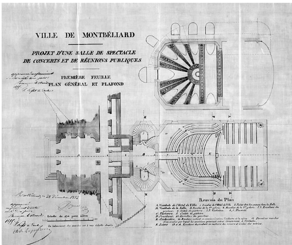
Projet de salle de spectacle (...) Plan général et plafond, 1854.
