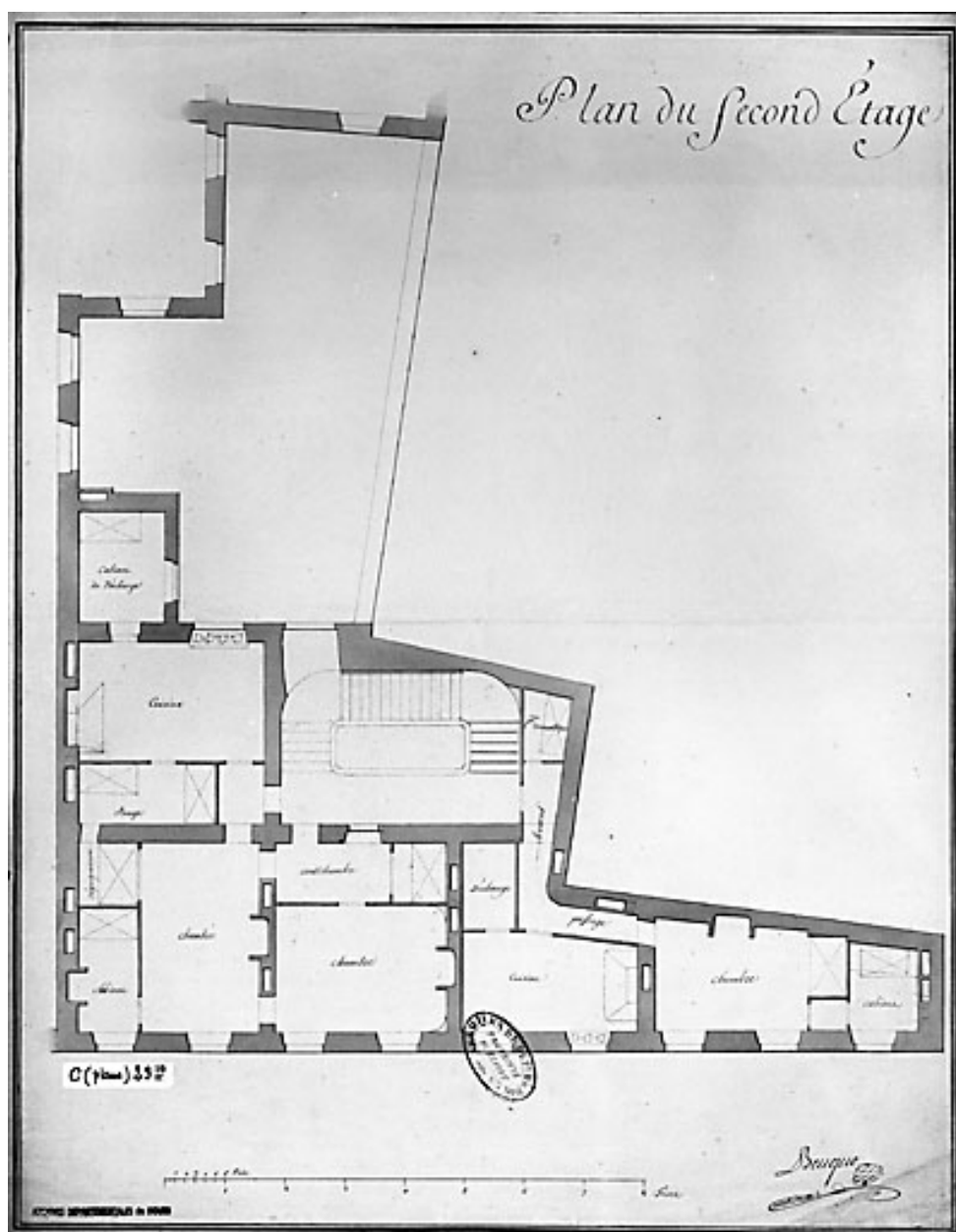
Plan du second étage.
