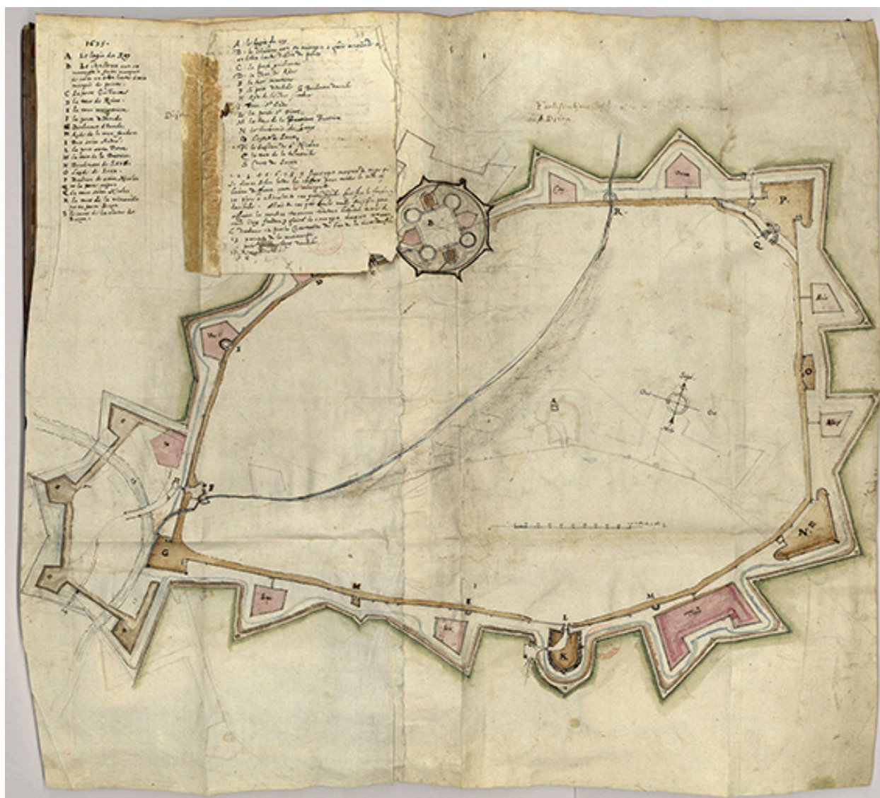
[Projet de renforcement des fortifications de Dijon]. 1635.
