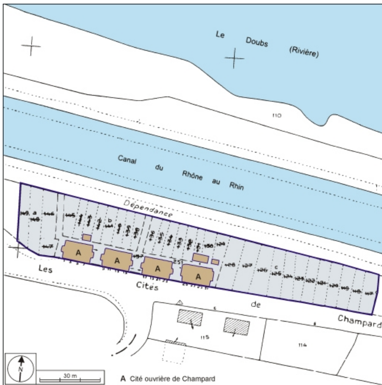
Plan de situation de la cité ouvrière de Champard. Extrait du plan cadastral, 1982, section AN, 1:1000.
