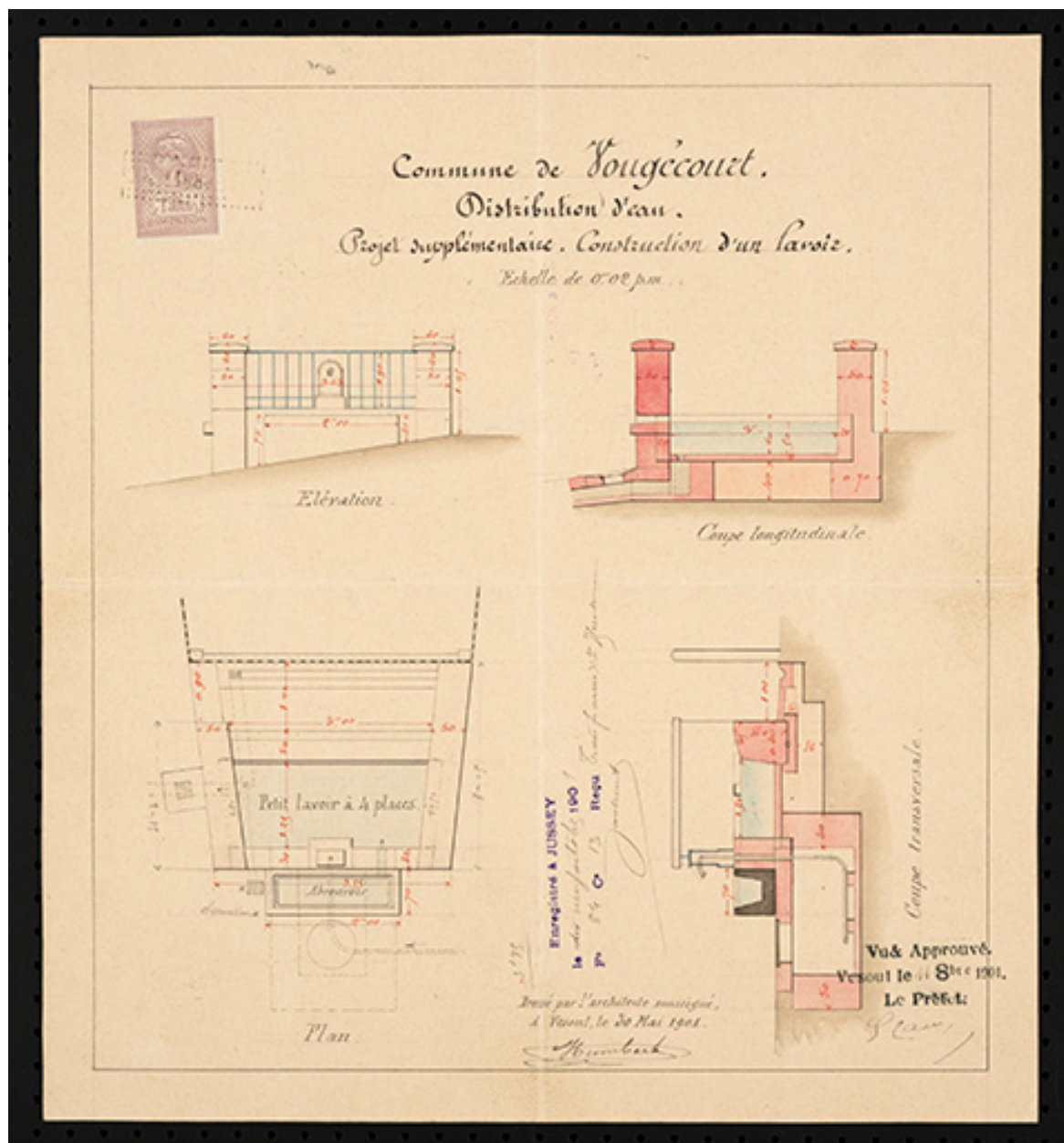
Distribution en eau, construction d'un lavoir. [plan] 1901
