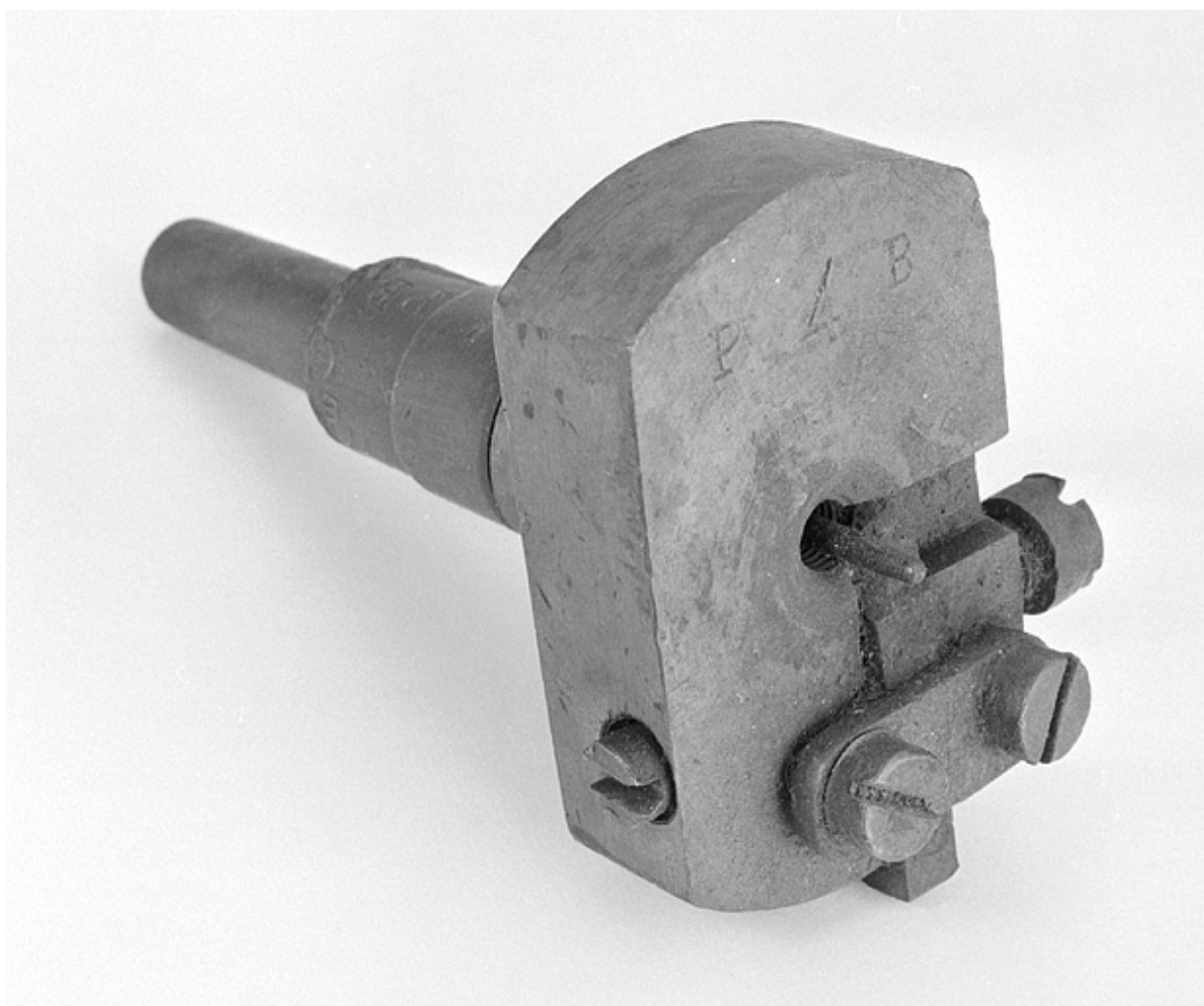
Détail d'un des outils de coupe.
