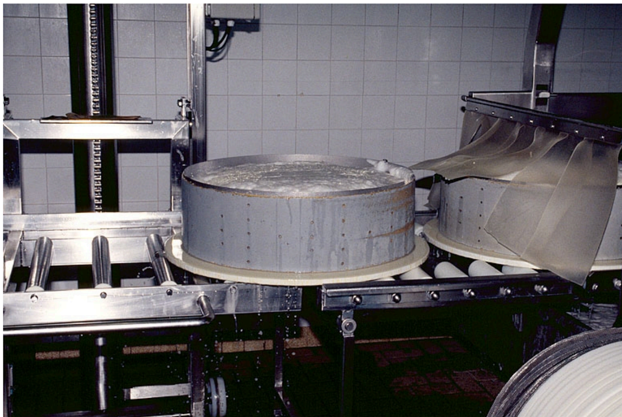
Moules remplies de caillé sortant du soutirage sous vide.
