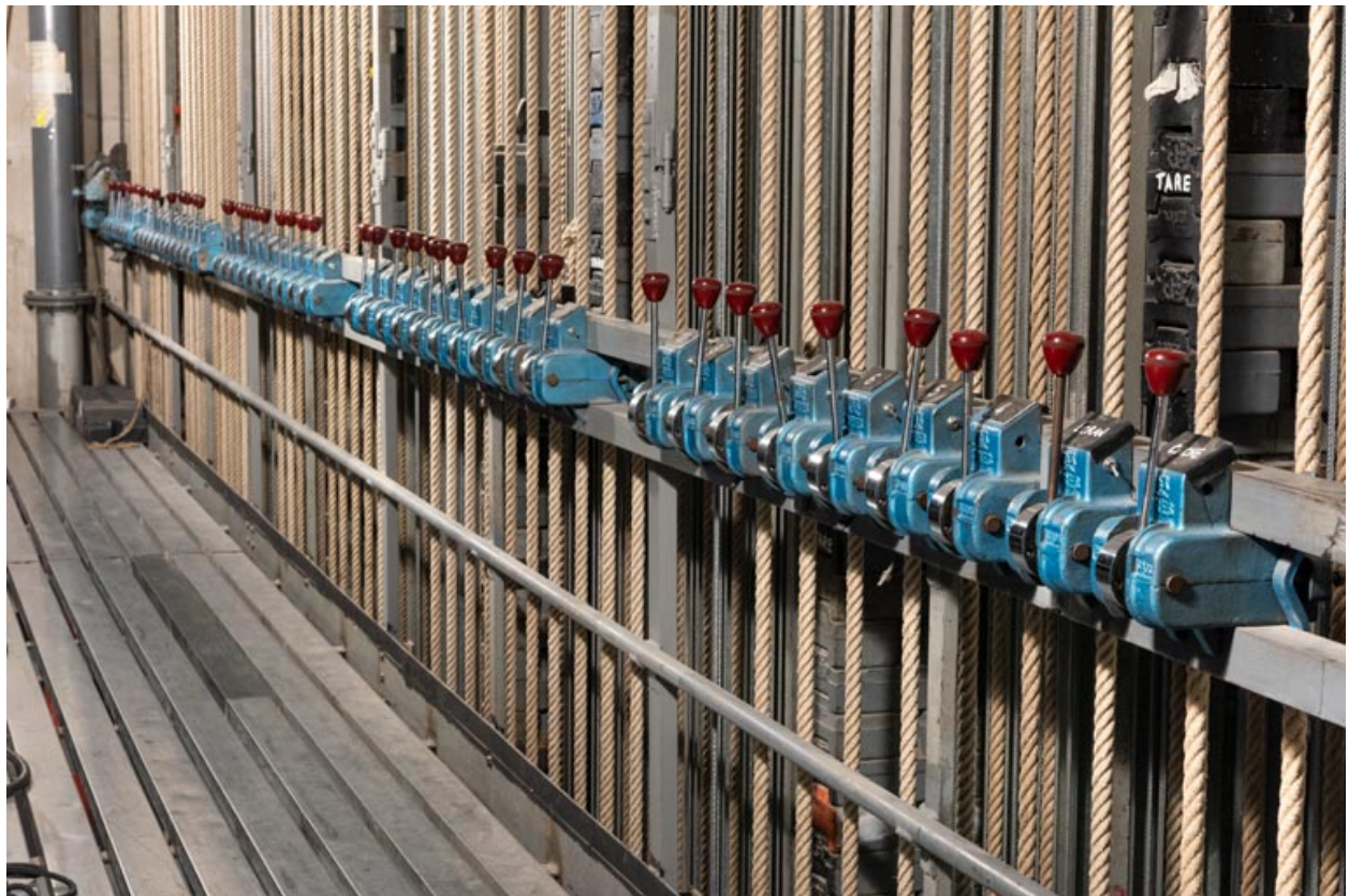
Maison de la culture, grande salle : freins à levier des équipes contrebalancées, sur la passerelle de commande (vue rapprochée).
